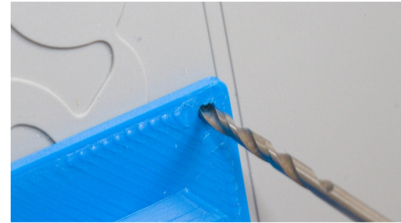
Abbildung 11: Bohren von Löchern für das Sensormodul
