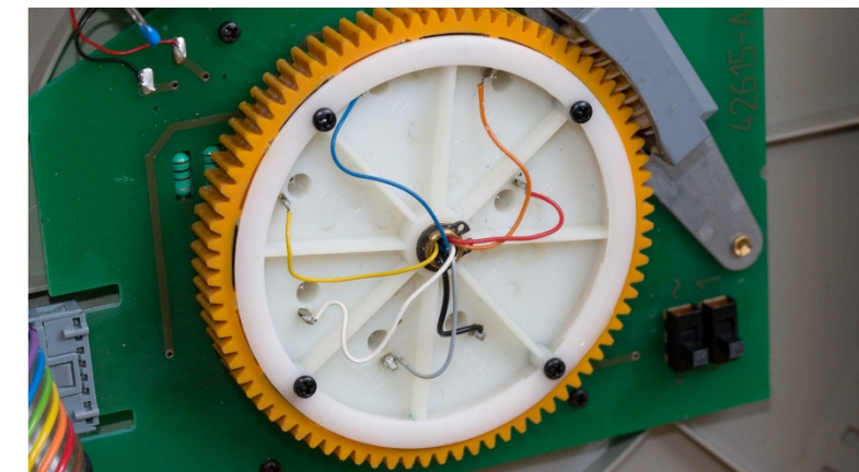
Abbildung 4: Scheibe mit Schleifkontakten
