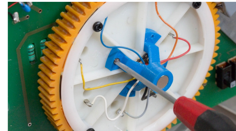
Abbildung 7: Magnethalter festschrauben
