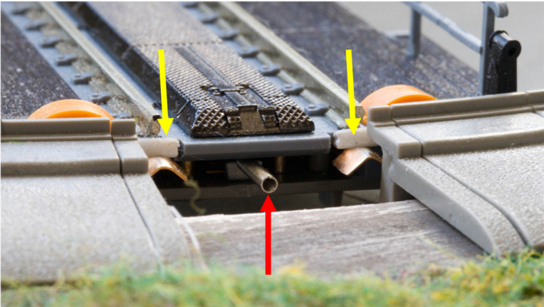
Abbildung 17 Gelb: Federkontakte mit Polystyrolstücken blockiert. Rot: Die in Abschnitt 3.3 beschriebene Feder
